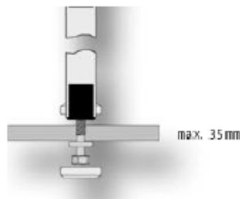
Montage der untersten Ablage (Ebene)
